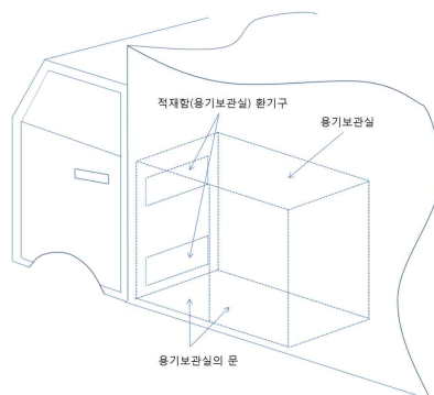
그림 2-2 적재함(용기보관실)에 환기구 설치
