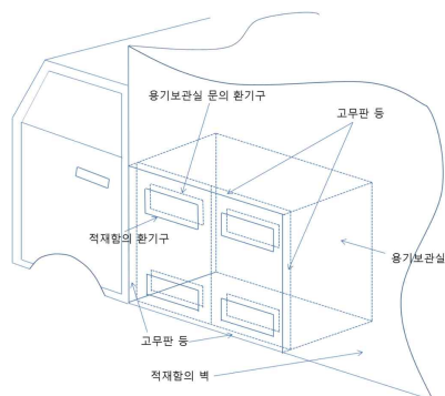
그림 2-1 용기보관실 문에 환기구 설치
